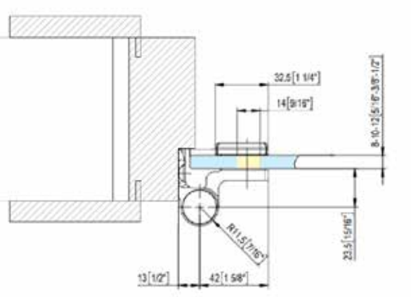
Sezione cerniera con stipite in legno Hinge with jamb wood section
