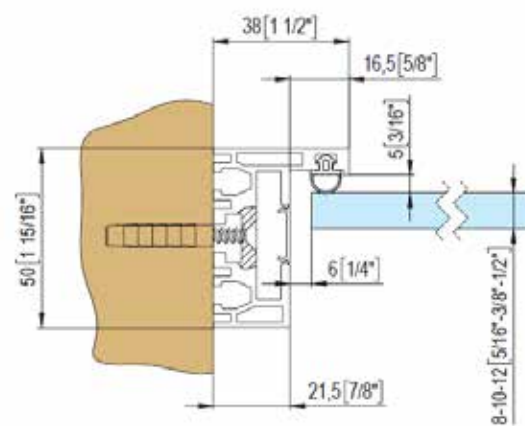
Sezione profilo di battuta in alluminio Aluminum stop profile section
