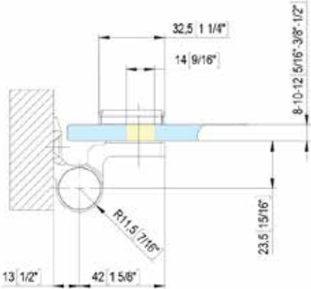
Sezione cerniera a parete Wall hinge section
